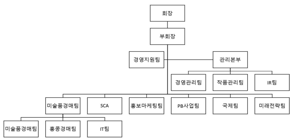
그림 07. 동사의 지배구조
